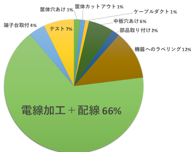
図1 制御盤製造における工数分析（ドイツにおける産学連携による調査）
