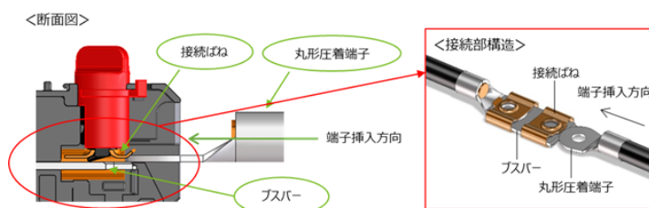
丸端子用の接続例
