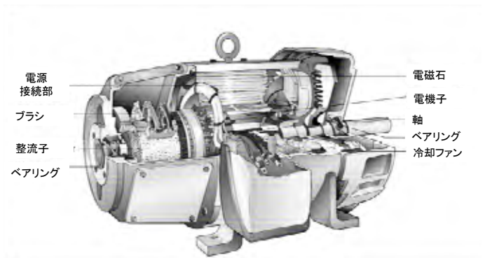
直流電動機
