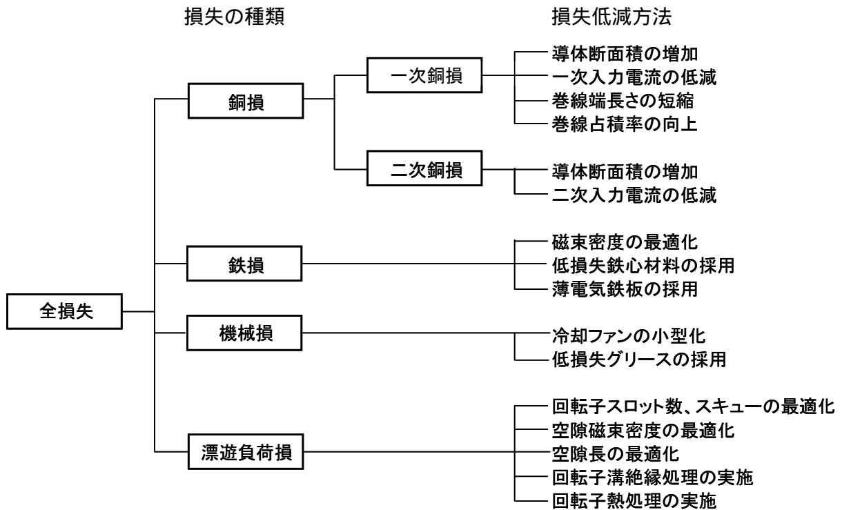
図4 電動機の損失発生に対する改善策
