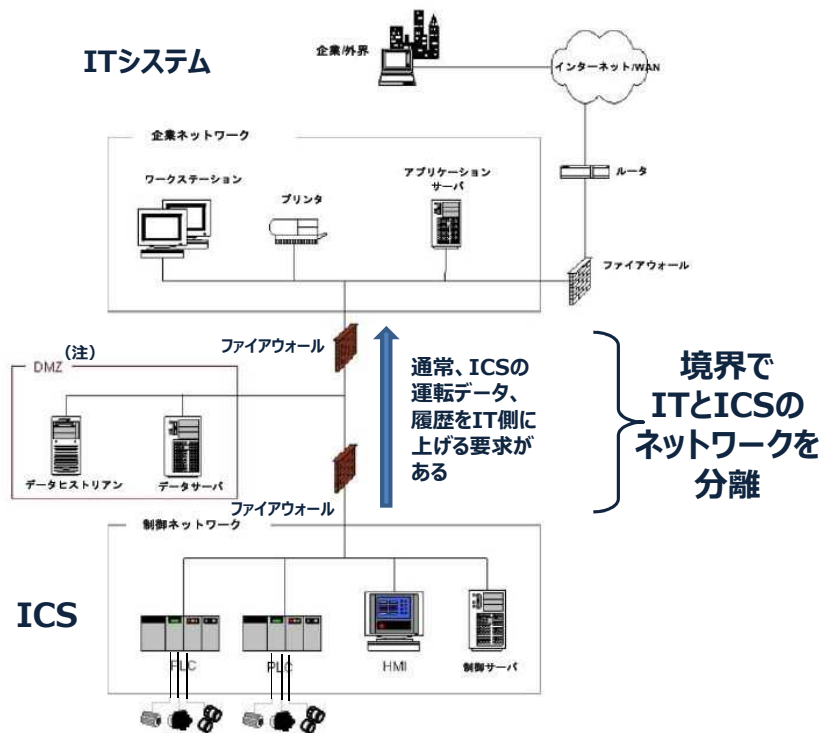
図. ICSセキュリティアーキテクチャ 出典：SP 800-82 Ver.2
