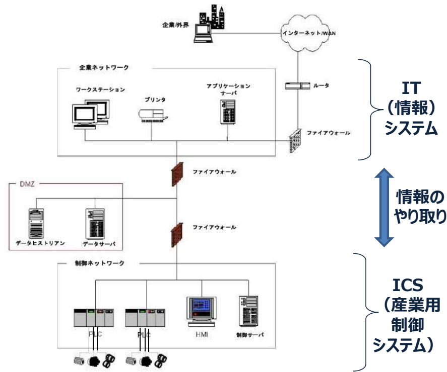
図. 情報（IT）システム と産業用制御システム（ICS） 出典：SP 800-82 Ver.2
