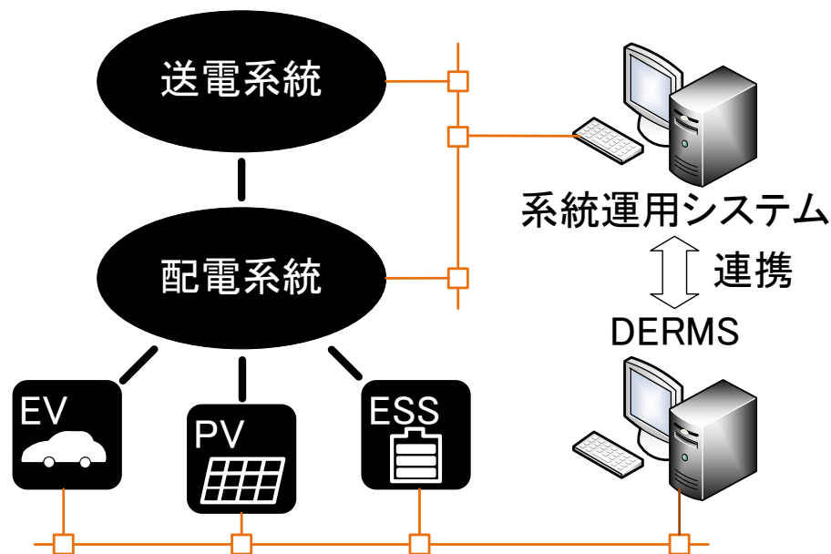
DERMSを用いた分散型電源管理の構成例
