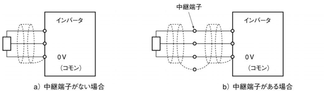
図9 シールド線の処理
