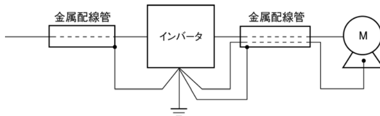
図8 金属配線管の接地
