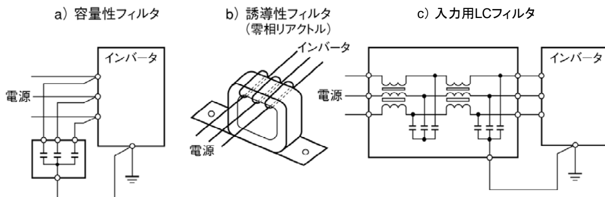
図10 各種フィルタ及び接続法
