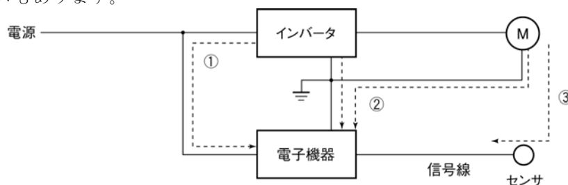
図3 伝導ノイズ
