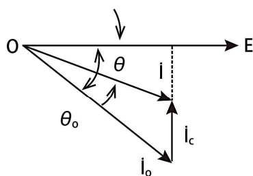
(a) ベクトル図
